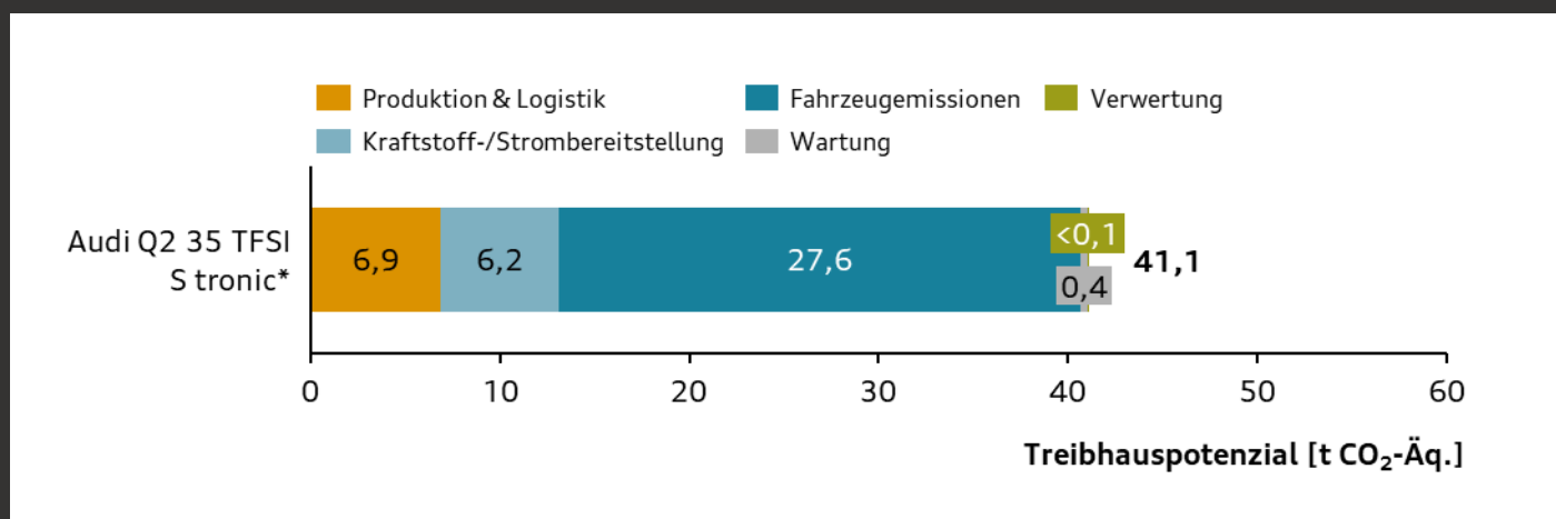
Abbildung 2: Treibhauspotenzial des Audi Q2 35 TFSI S tronic* über den gesamten Lebenszyklus
