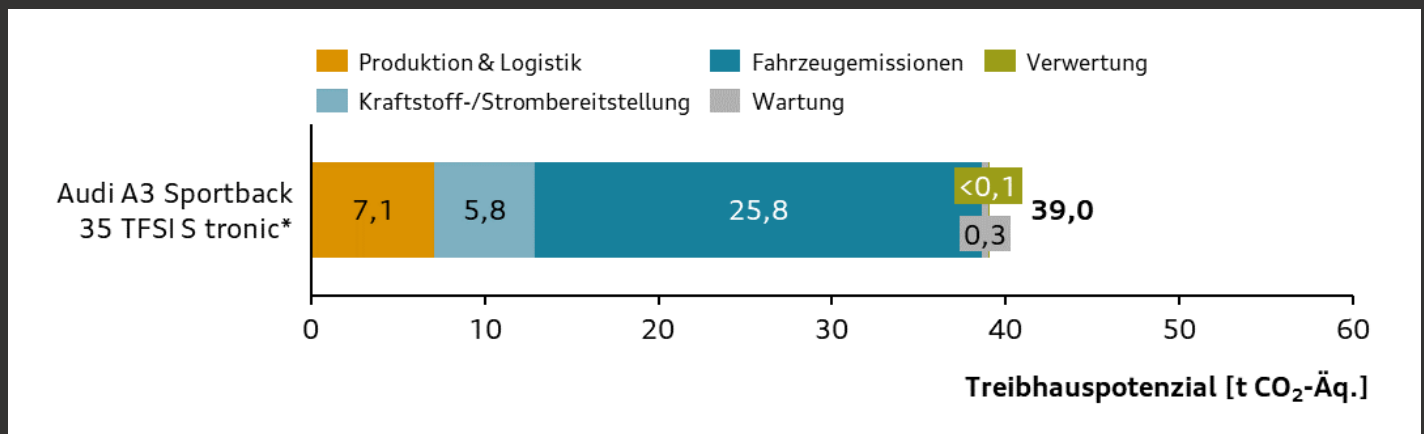
Abbildung 2: Treibhauspotenzial des Audi A3 Sportback 35 TFSI S tronic* über den gesamten Lebenszyklus
